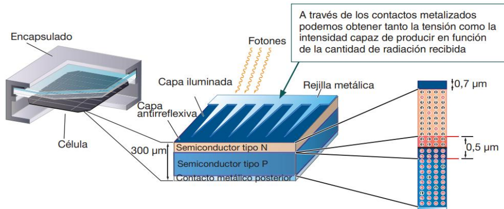
Figura 1, estructura de una célula fotovoltaica.
